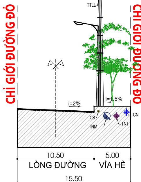
MẶT CẮT 5 - 5 (LỘ GIỚI 15,5M)
