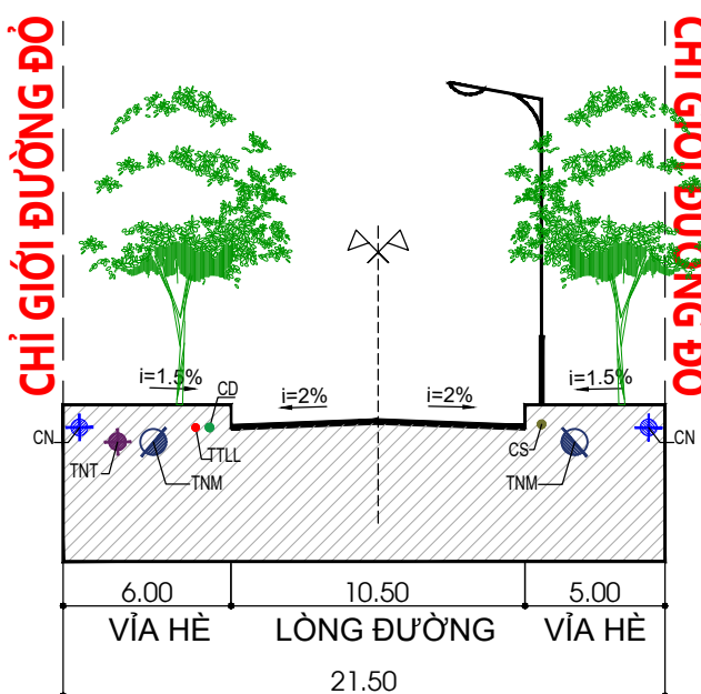
MẶT CẮT 4 - 4 (LỘ GIỚI 21,5M)
