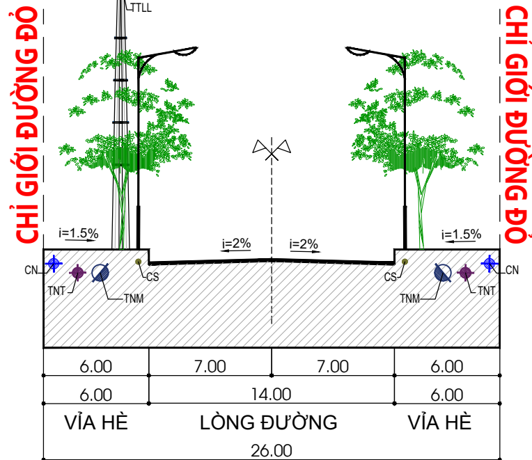
MẶT CẮT 1 - 1 (LỘ GIỚI 26M)
