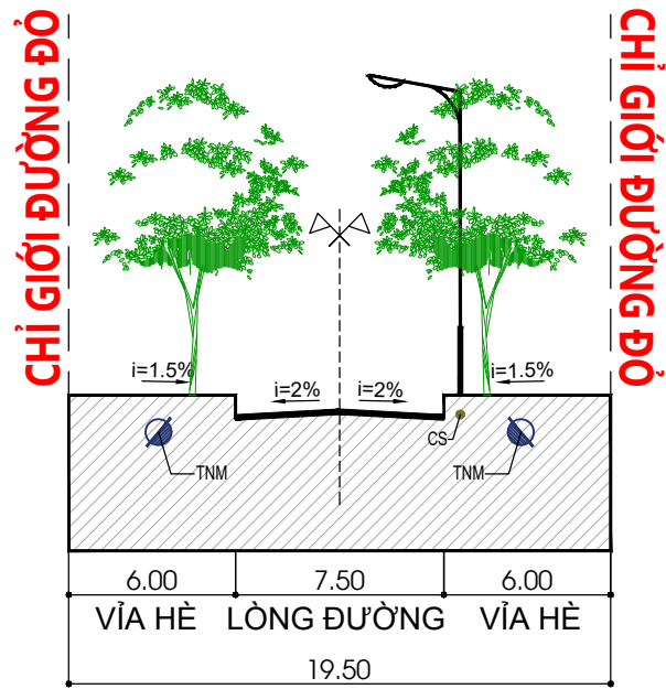
MẶT CẮT 2 - 2 (LỘ GIỚI 19,5M)
