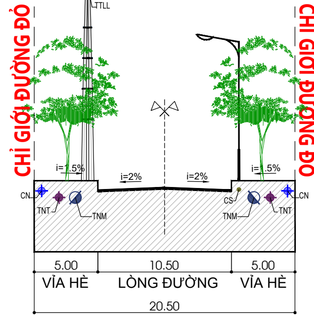
MẶT CẮT 3 - 3 (LỘ GIỚI 21,5M)
