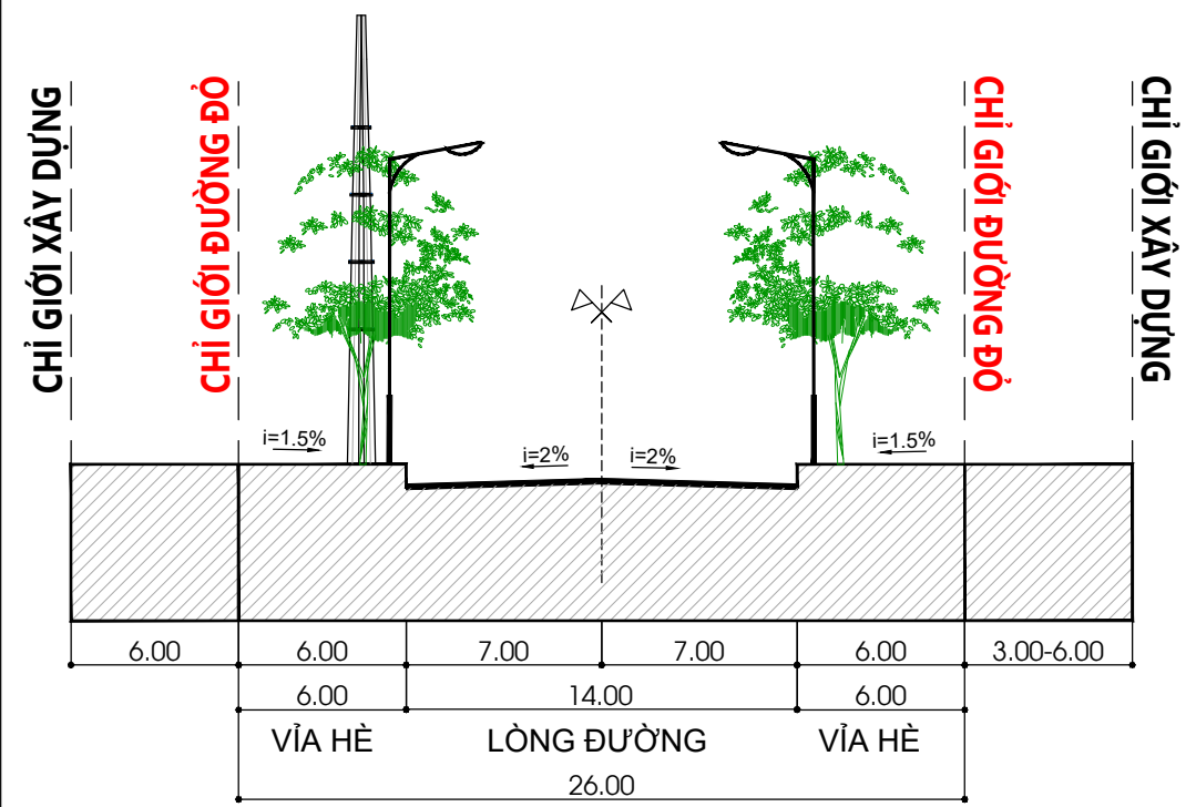
MẶT CẮT 1 - 1 (LỘ GIỚI 26M)
