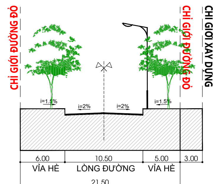
MẶT CẮT 4 - 4 (LỘ GIỚI 21,5M)
