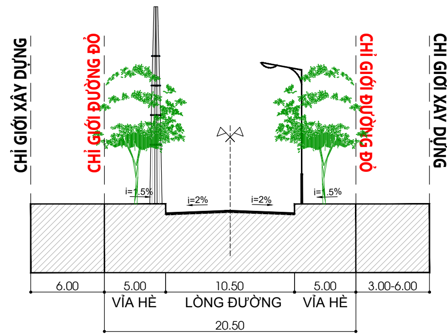
MẶT CẮT 3 - 3 (LỘ GIỚI 21,5M)
