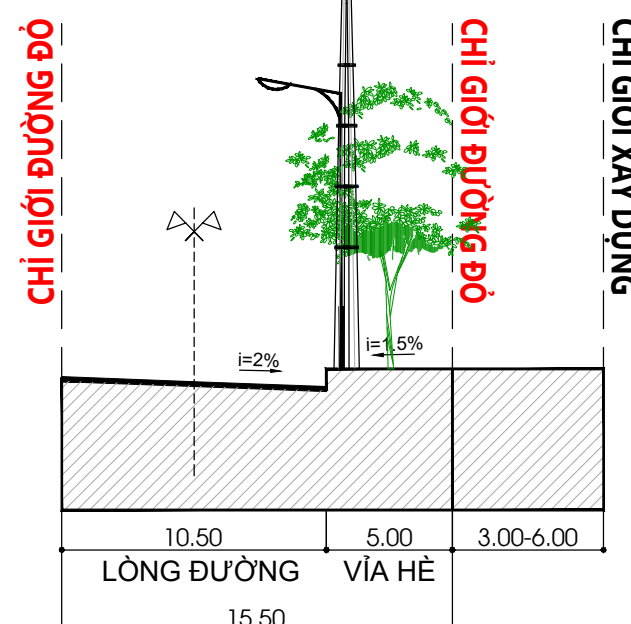
MẶT CẮT 5 - 5 (LỘ GIỚI 15,5M)
