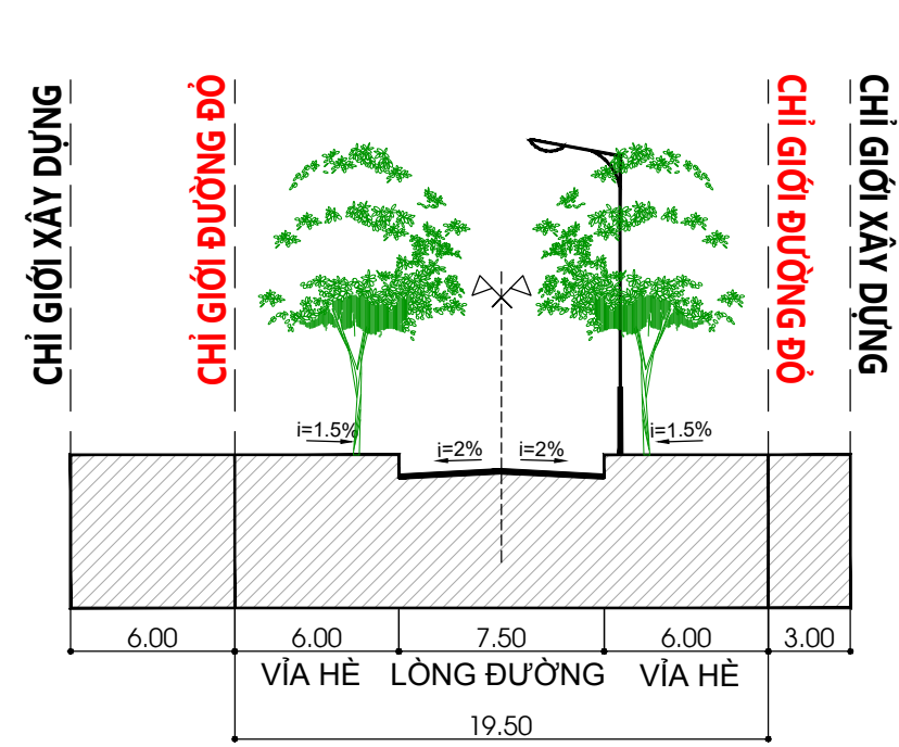
MẶT CẮT 2 - 2 (LỘ GIỚI 19,5M)
