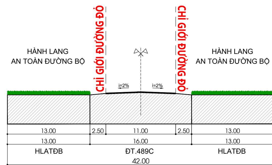
MẶT CẮT TUYẾN NHÁNH 489C (LỘ GIỚI 42M)
