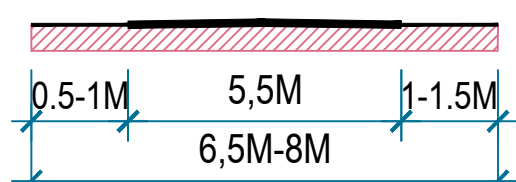
MẶT CẮT 3 - 3 (TRỤC XÃ 1, ĐOẠN TỪ HL.XUÂN THỦY NAM ĐIỂN ĐẾN CẦU ĐỒI)
