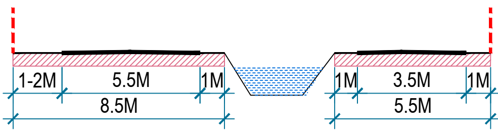
MẶT CẮT 2 - 2
