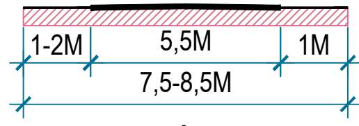
MẶT CẮT 1 - 1 (HL. XUÂN THỦY - NAM ĐIỂN)
