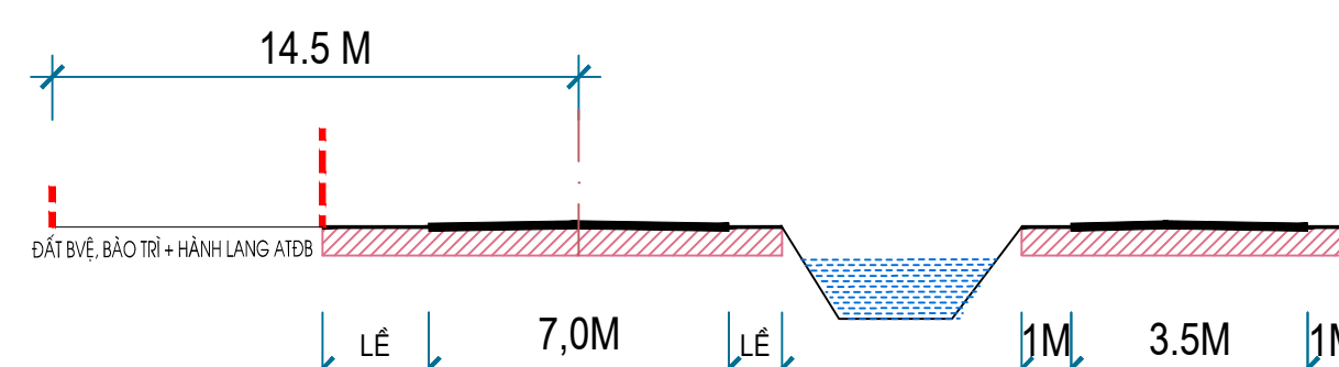
MẶT CẮT 2-2
