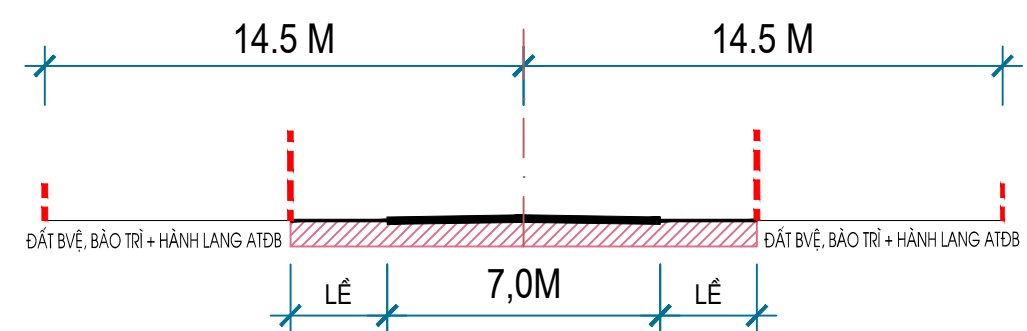
MẶT CẮT 1-1 (HL. XUÂN THỦY - NAM ĐIỆN)
