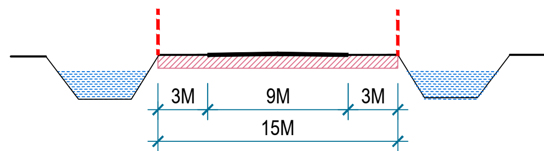
MẶT CẮT 3-3
